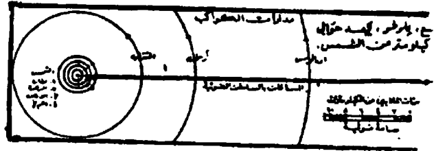
أبعاد الكواكب عن الشمس
